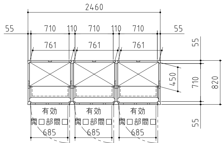
平面図
